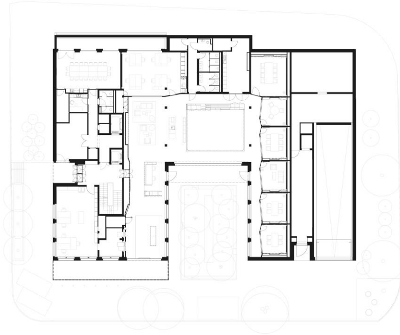
Bürräume: 3. Obergeschoss
